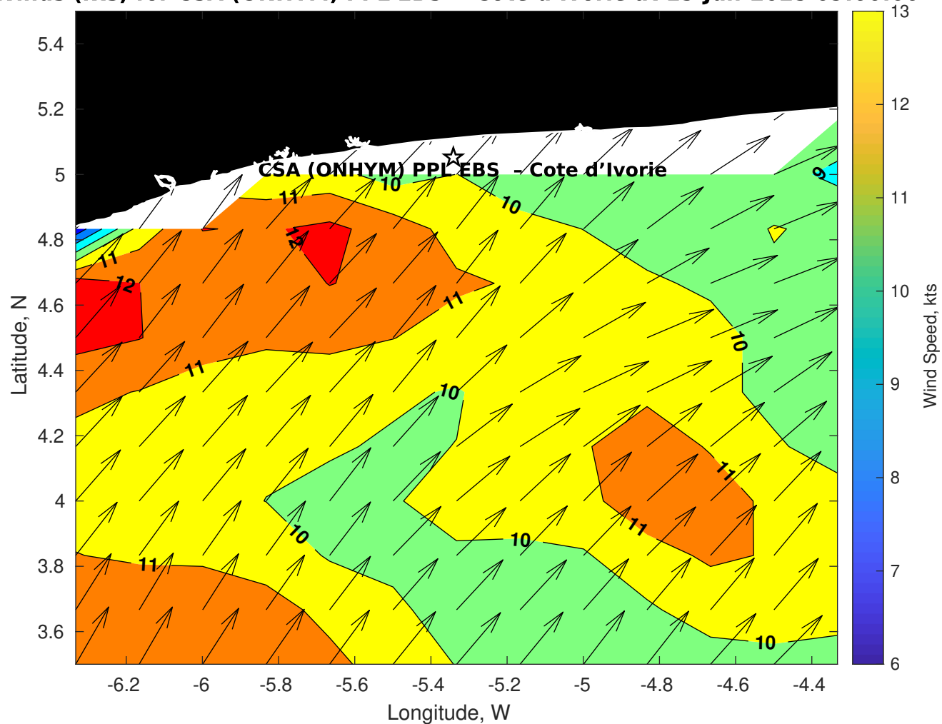
Winds (kts) for CSA (ONHYM) PPL EBS - Cote d'Ivoire at 15-Jun-2025 09:00:00
