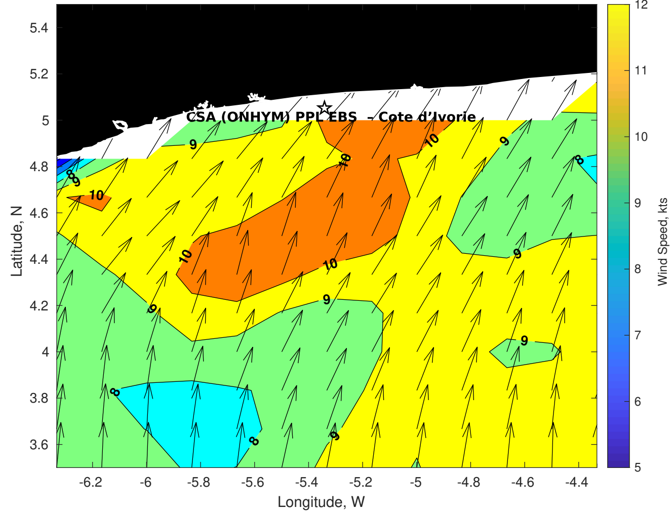
Winds (kts) for CSA (ONHYM) PPL EBS - Cote d'Ivoire at 25-Jul-2025 21:00:00
