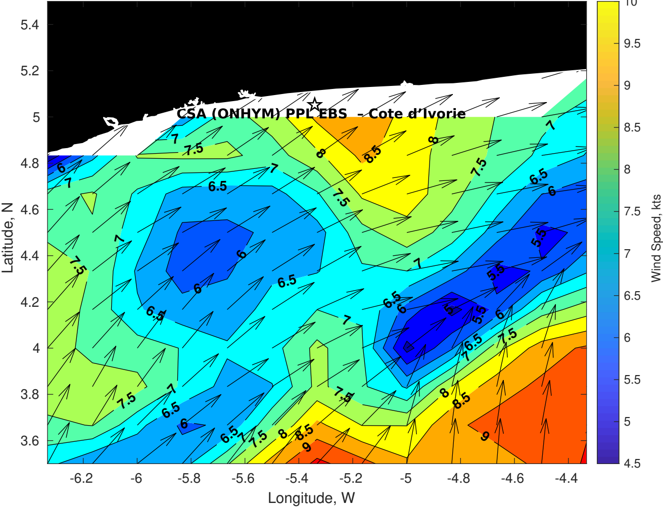
Winds (kts) for CSA (ONHYM) PPL EBS - Cote d'Ivoire at 07-Sep-2025 09:00:00
