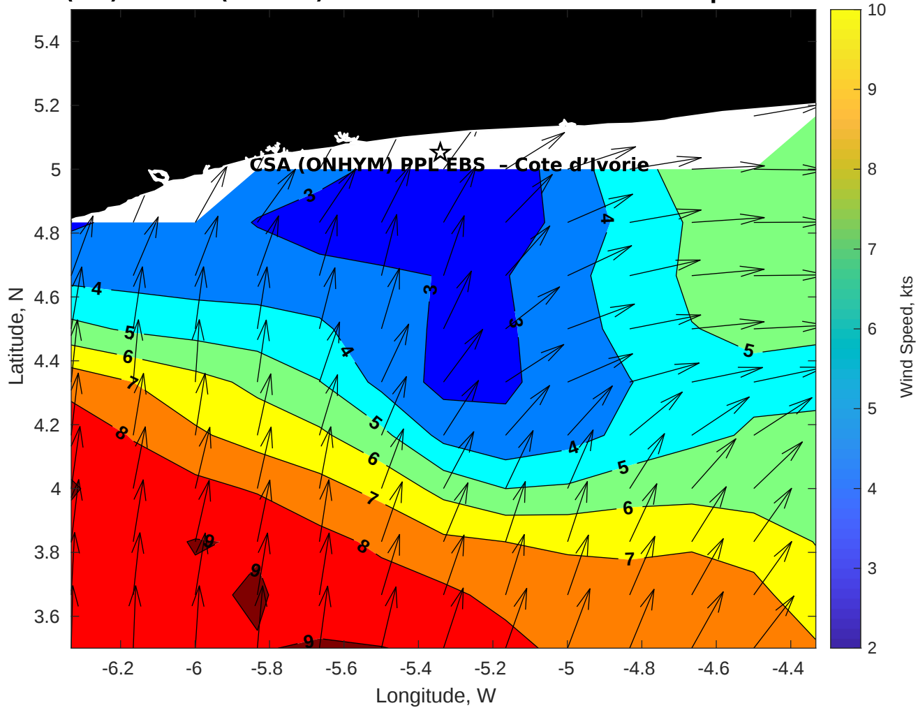
Winds (kts) for CSA (ONHYM) PPL EBS - Cote d'Ivoire at 15-Sep-2025 09:00:00
