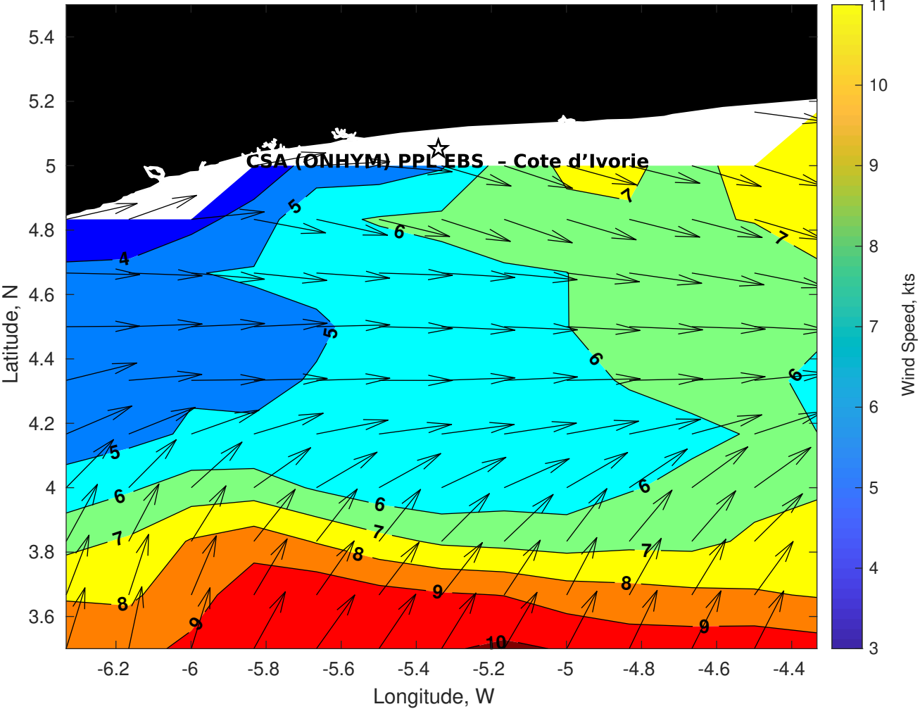
Winds (kts) for CSA (ONHYM) PPL EBS - Cote d'Ivoire at 25-Sep-2025 09:00:00
