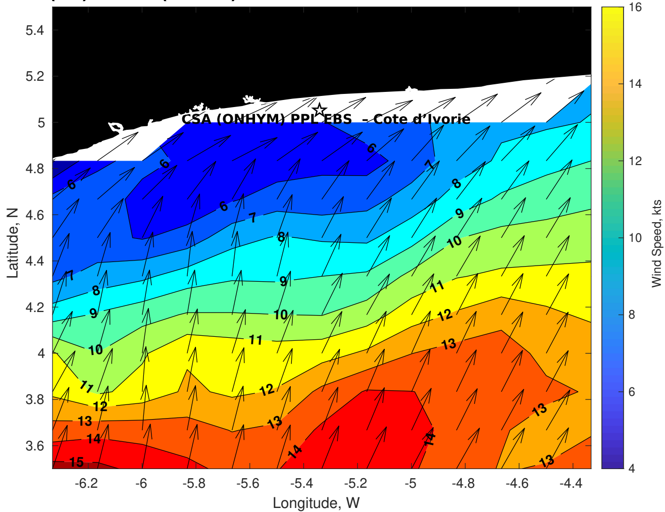
Winds (kts) for CSA (ONHYM) PPL EBS - Cote d'Ivoire at 05-Oct-2025 09:00:00
