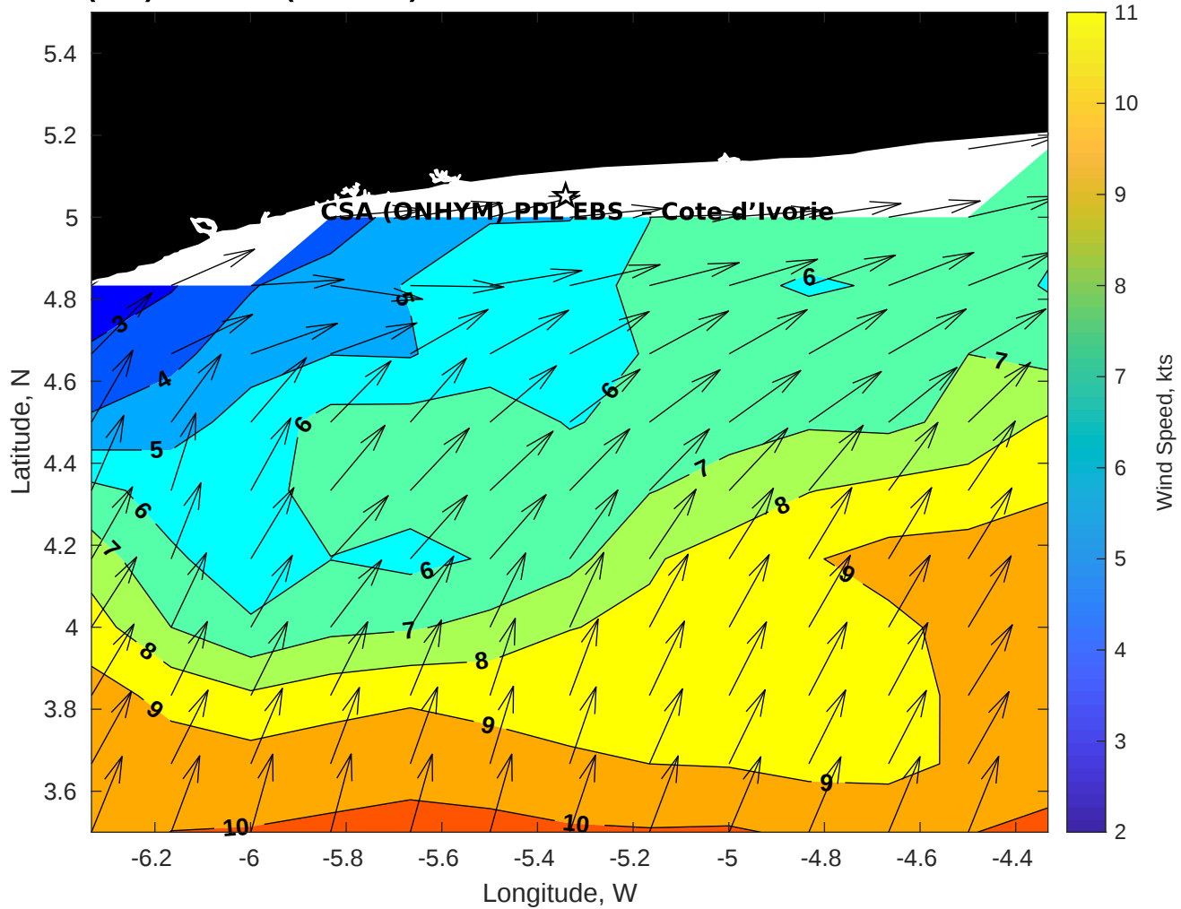
Winds (kts) for CSA (ONHYM) PPL EBS - Cote d'Ivoire at 06-Oct-2025 09:00:00
