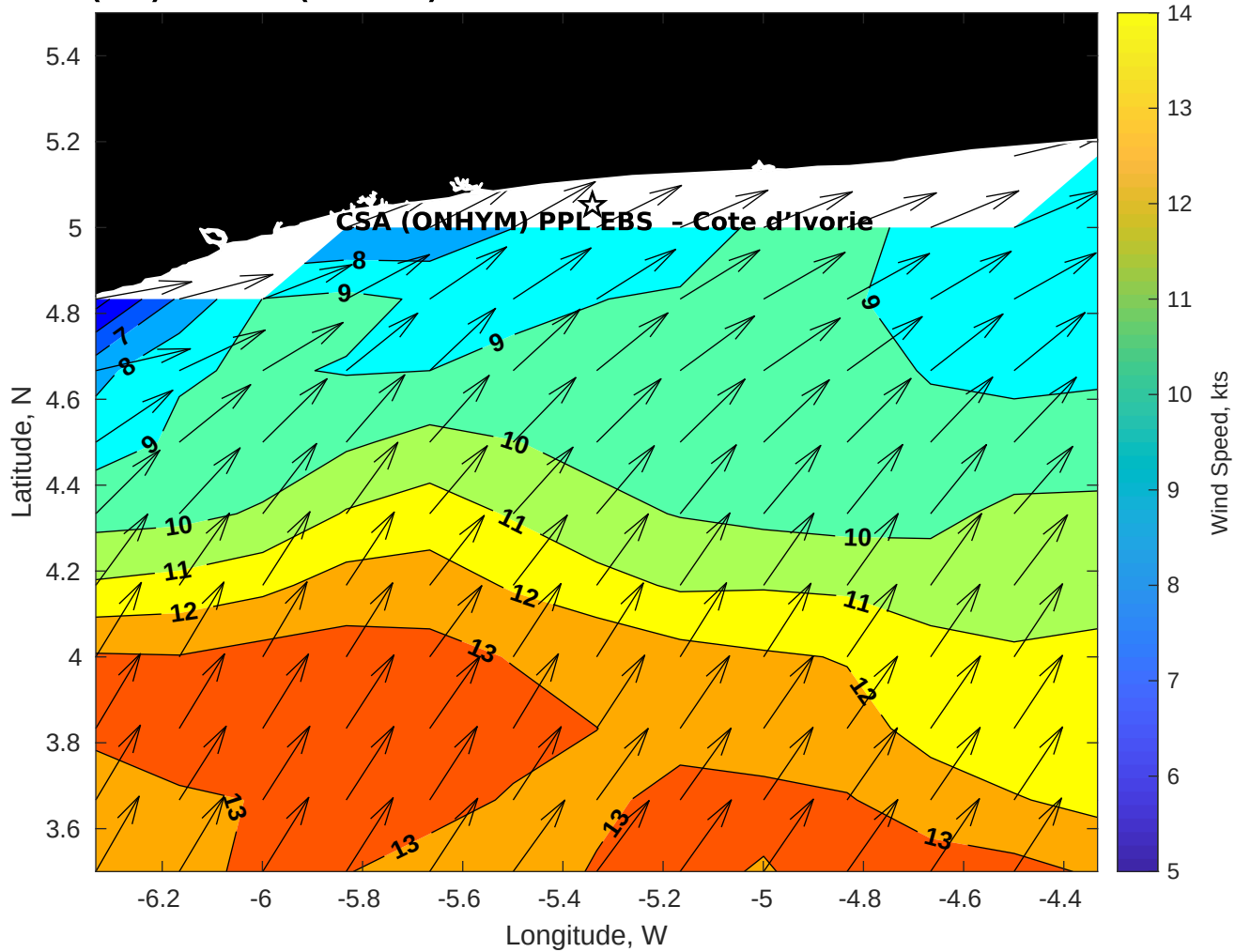
Winds (kts) for CSA (ONHYM) PPL EBS - Cote d'Ivoire at 14-Oct-2025 09:00:00
