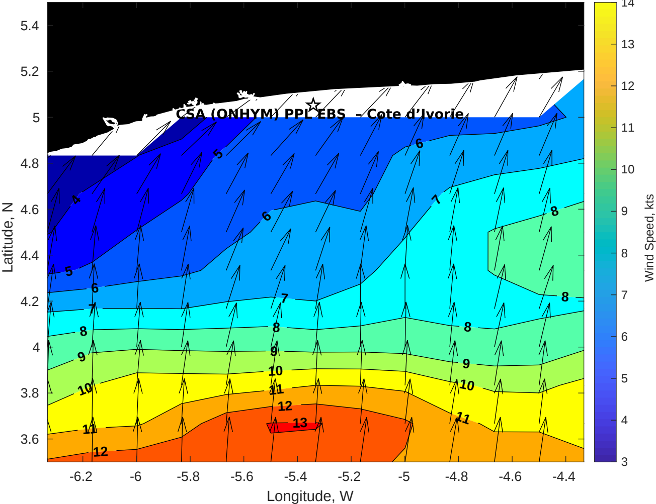
Winds (kts) for CSA (ONHYM) PPL EBS - Cote d'Ivoire at 16-Oct-2025 09:00:00
