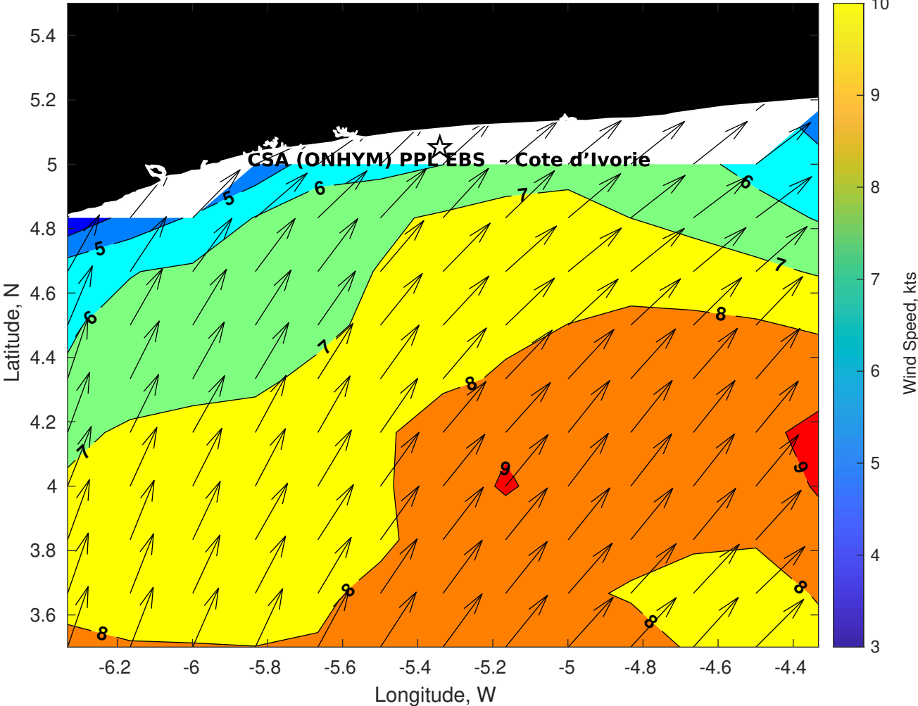
Winds (kts) for CSA (ONHYM) PPL EBS - Cote d'Ivoire at 19-Oct-2025 09:00:00
