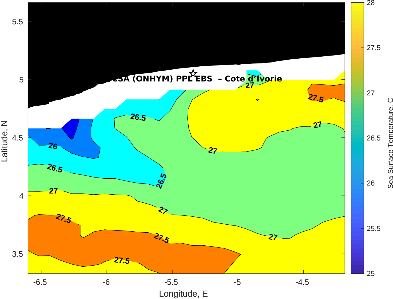
SST for CSA (ONHYM) PPL EBS - Cote d'Ivoire at 22-Oct-2025 00:00:00
