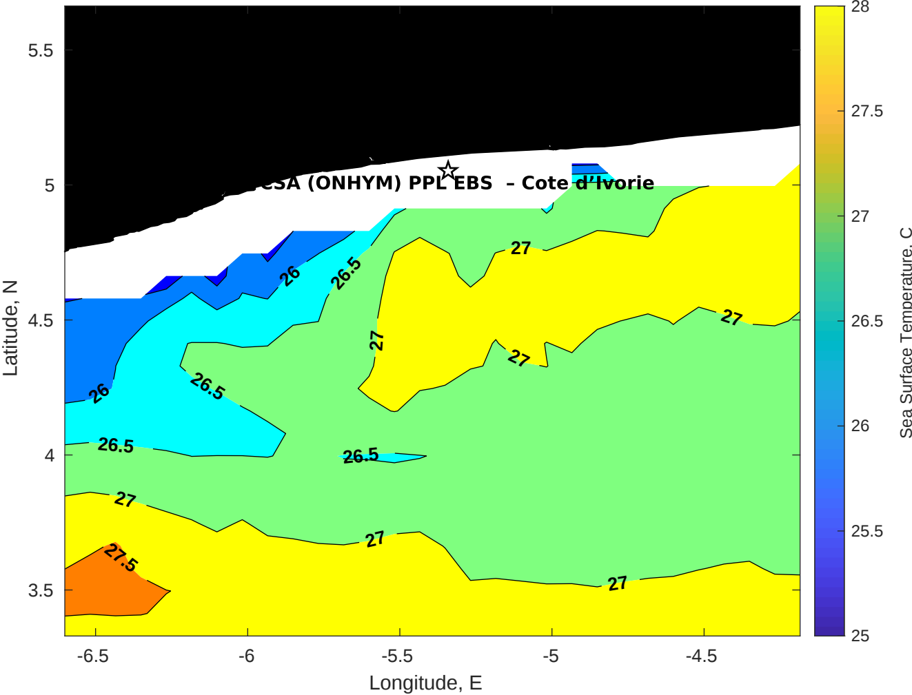
SST for CSA (ONHYM) PPL EBS - Cote d'Ivoire at 25-Oct-2025 00:00:00
