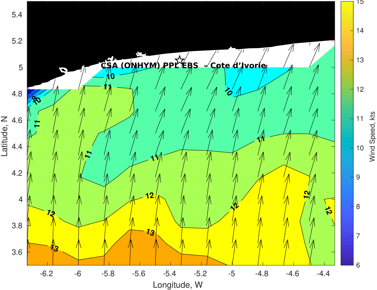
Winds (kts) for CSA (ONHYM) PPL EBS - Cote d'Ivoire at 01-Nov-2025 09:00:00
