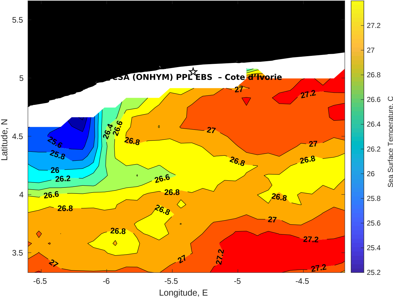
SST for CSA (ONHYM) PPL EBS - Cote d'Ivoire at 01-Nov-2025 00:00:00
