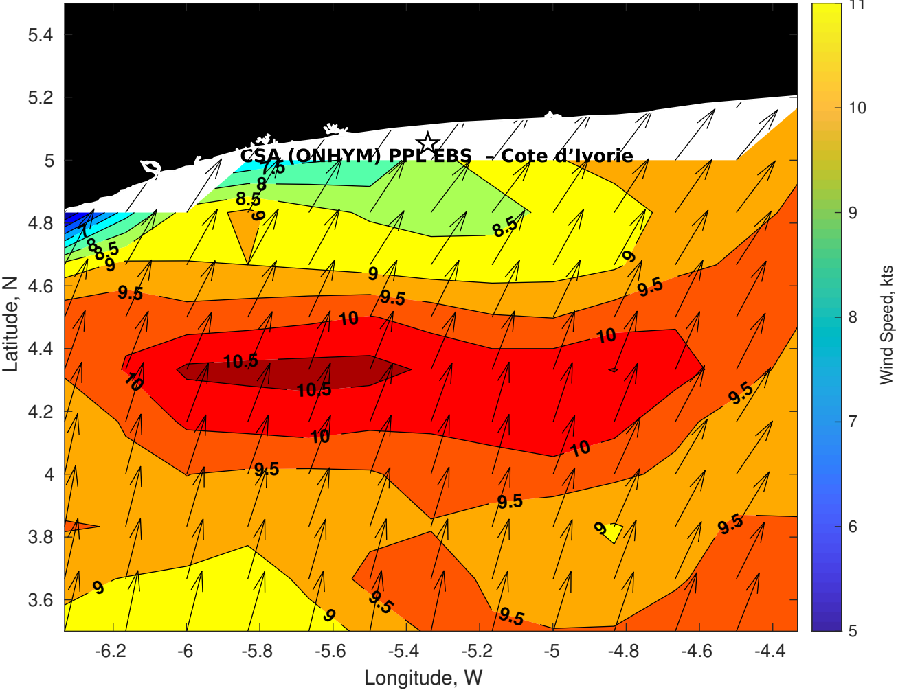
Winds (kts) for CSA (ONHYM) PPL EBS - Cote d'Ivoire at 02-Nov-2025 09:00:00
