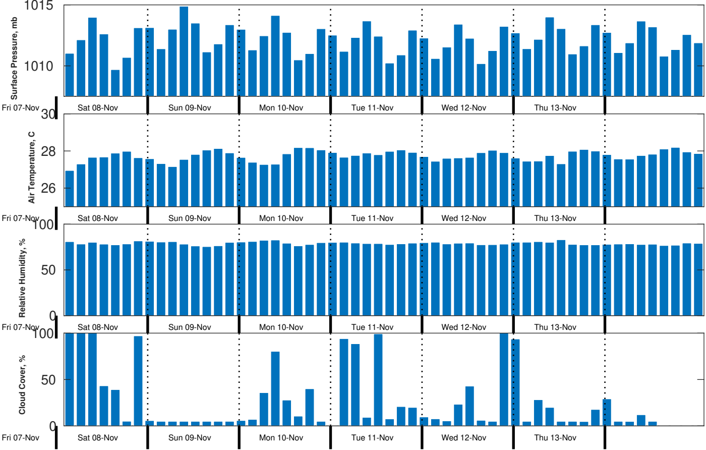
Met Forecast for CSA (ONHYM) PPL EBS - Cote d'Ivoire from 08-Nov-2025 00:00:00 to 15-Nov-2025 00:00:00
