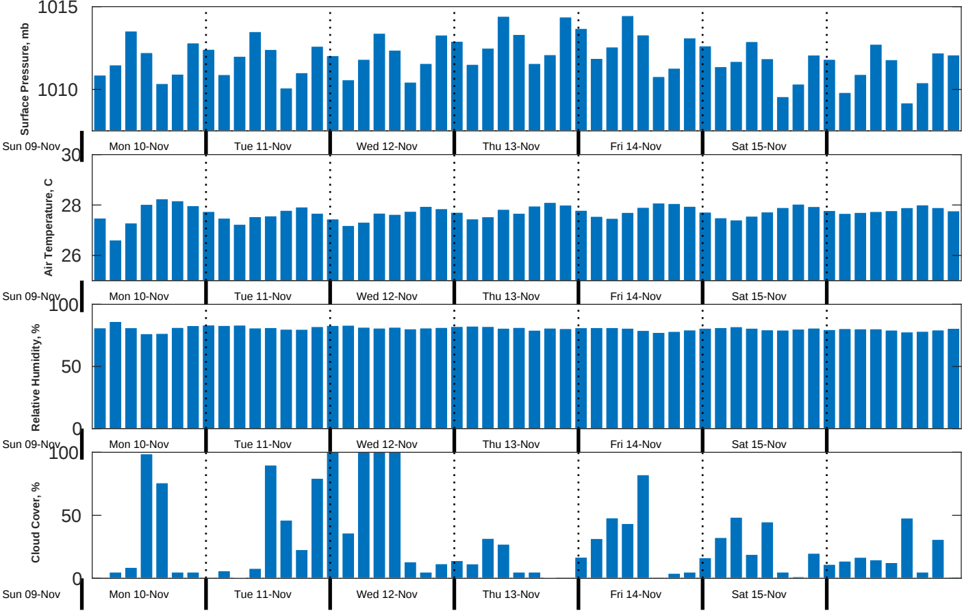
Met Forecast for CSA (ONHYM) PPL EBS - Cote d'Ivoire from 10-Nov-2025 00:00:00 to 17-Nov-2025 00:00:00
