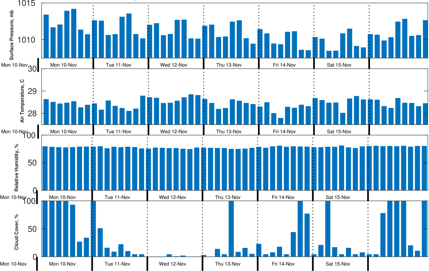
Met Forecast for Gyre from 10-Nov-2025 20:00:00 to 17-Nov-2025 20:00:00
