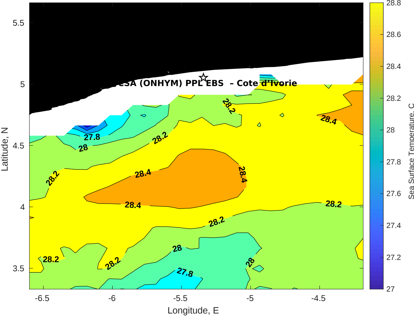
SST for CSA (ONHYM) PPL EBS - Cote d'Ivoire at 21-Nov-2025 00:00:00
