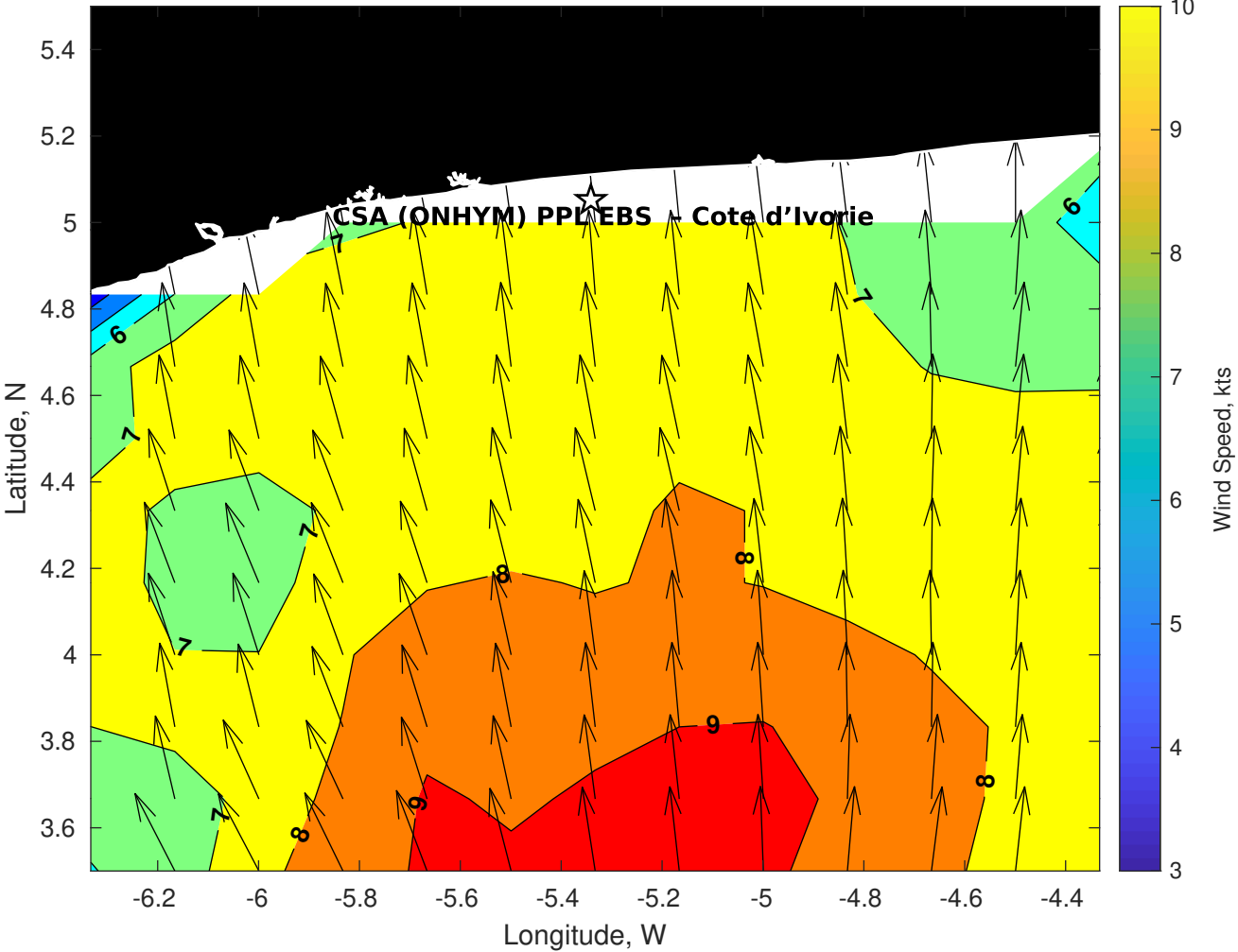
GFS Winds (kts) for CSA (ONHYM) PPL EBS - Cote d'Ivoire at 22-Nov-2025 09:00:00
