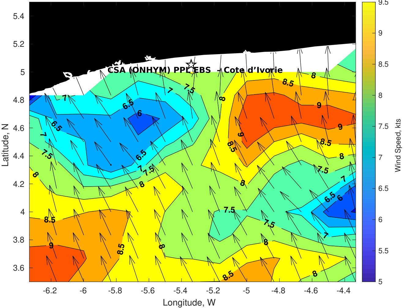
GFS Winds (kts) for CSA (ONHYM) PPL EBS - Cote d'Ivoire at 23-Nov-2025 09:00:00
