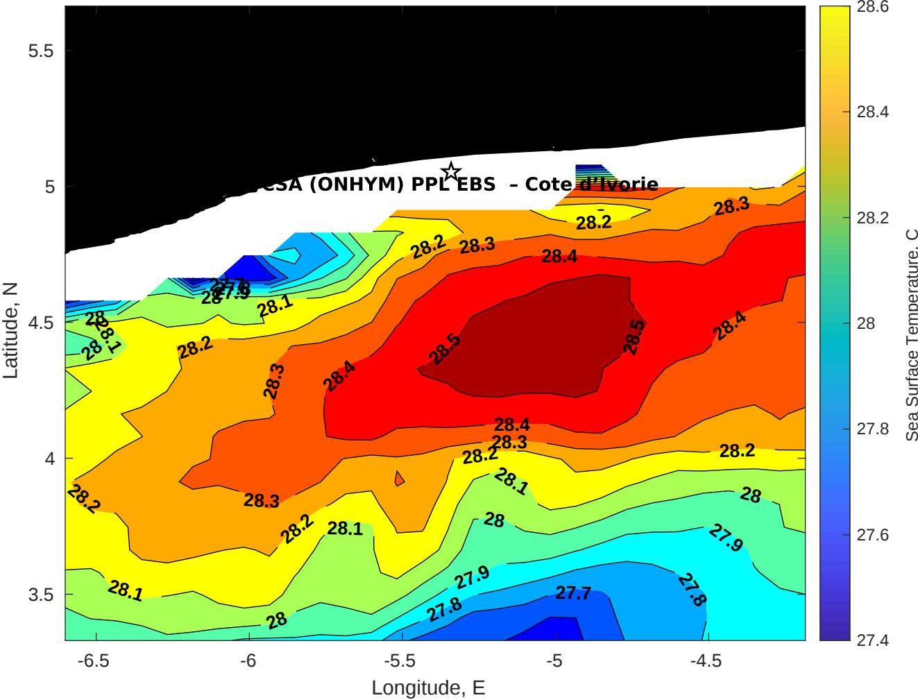
SST for CSA (ONHYM) PPL EBS - Cote d'Ivoire at 24-Nov-2025 00:00:00
