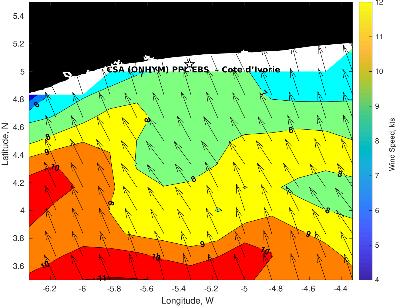
GFS Winds (kts) for CSA (ONHYM) PPL EBS - Cote d'Ivoire at 25-Nov-2025 09:00:00
