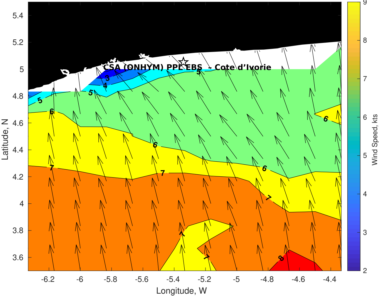
GFS Winds (kts) for CSA (ONHYM) PPL EBS - Cote d'Ivoire at 26-Nov-2025 09:00:00
