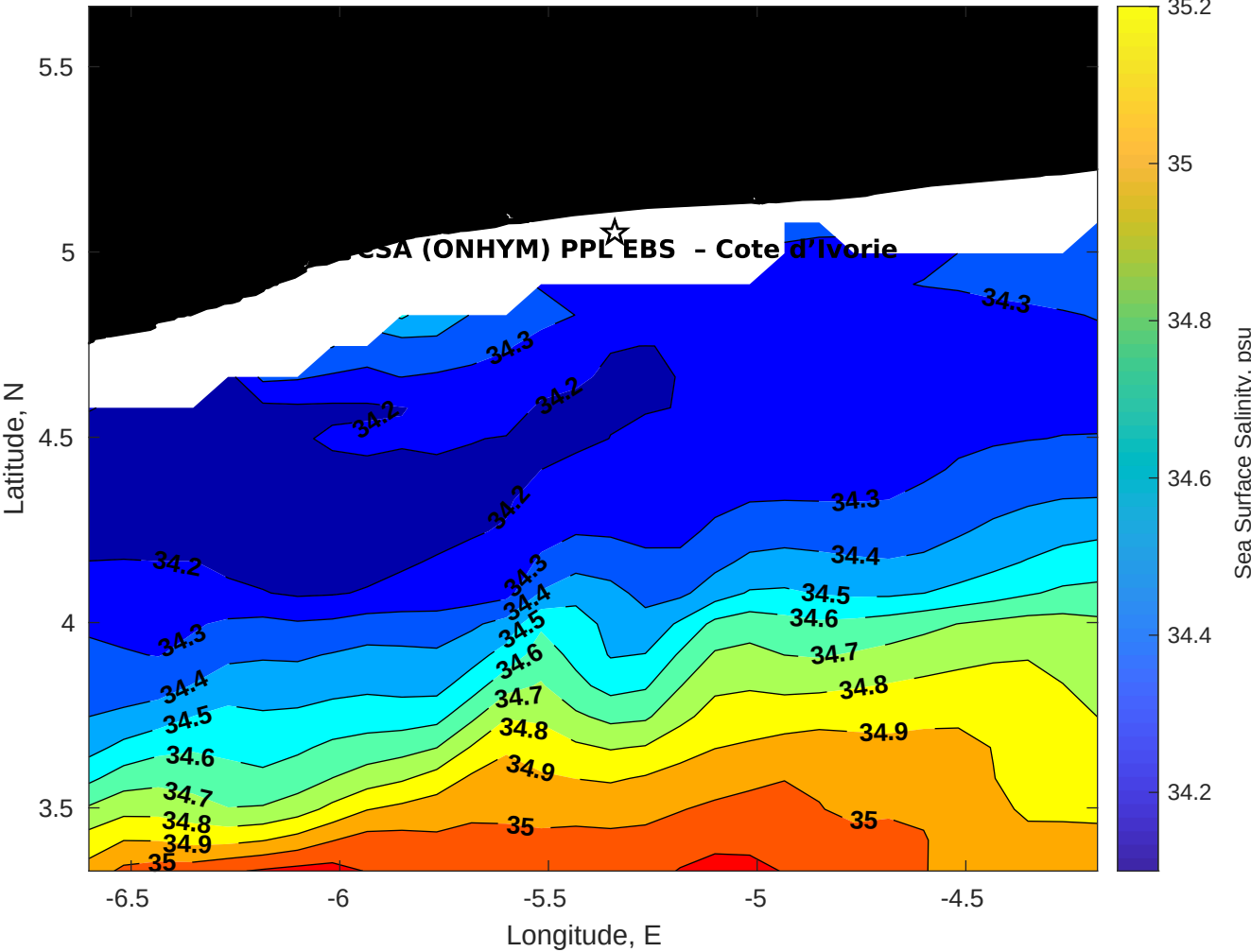
Surface Salinity for CSA (ONHYM) PPL EBS - Cote d'Ivoire at 27-Nov-2025 00:00:00
