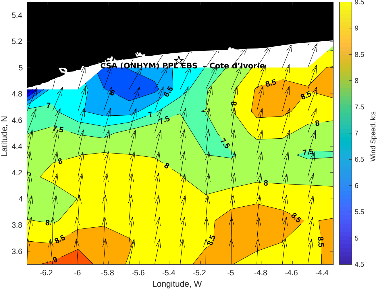
GFS Winds (kts) for CSA (ONHYM) PPL EBS - Cote d'Ivoire at 28-Nov-2025 09:00:00
