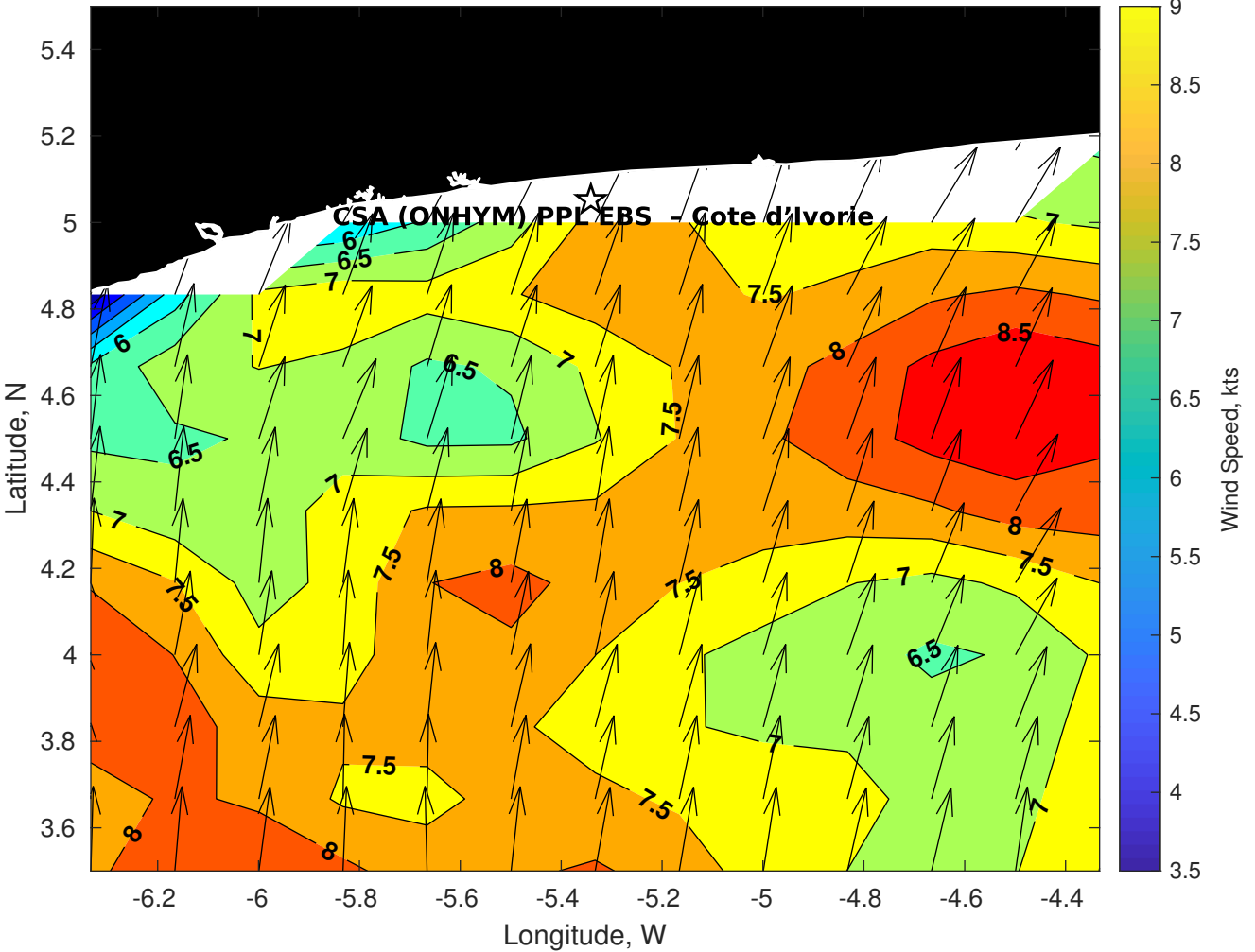
GFS Winds (kts) for CSA (ONHYM) PPL EBS - Cote d'Ivoire at 30-Nov-2025 09:00:00
