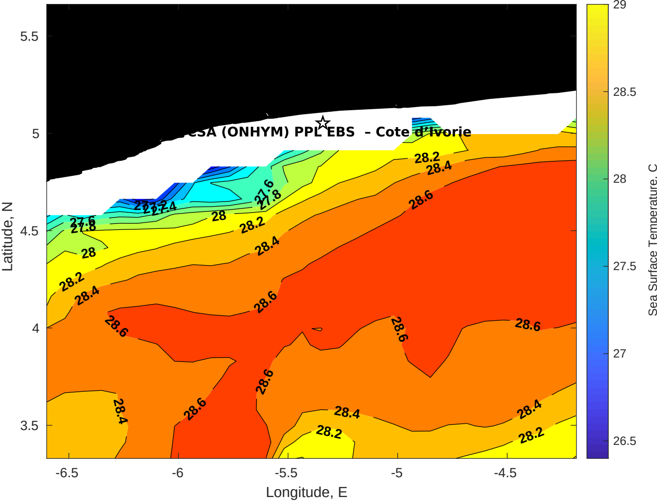
SST for CSA (ONHYM) PPL EBS - Cote d'Ivoire at 04-Dec-2025 00:00:00
