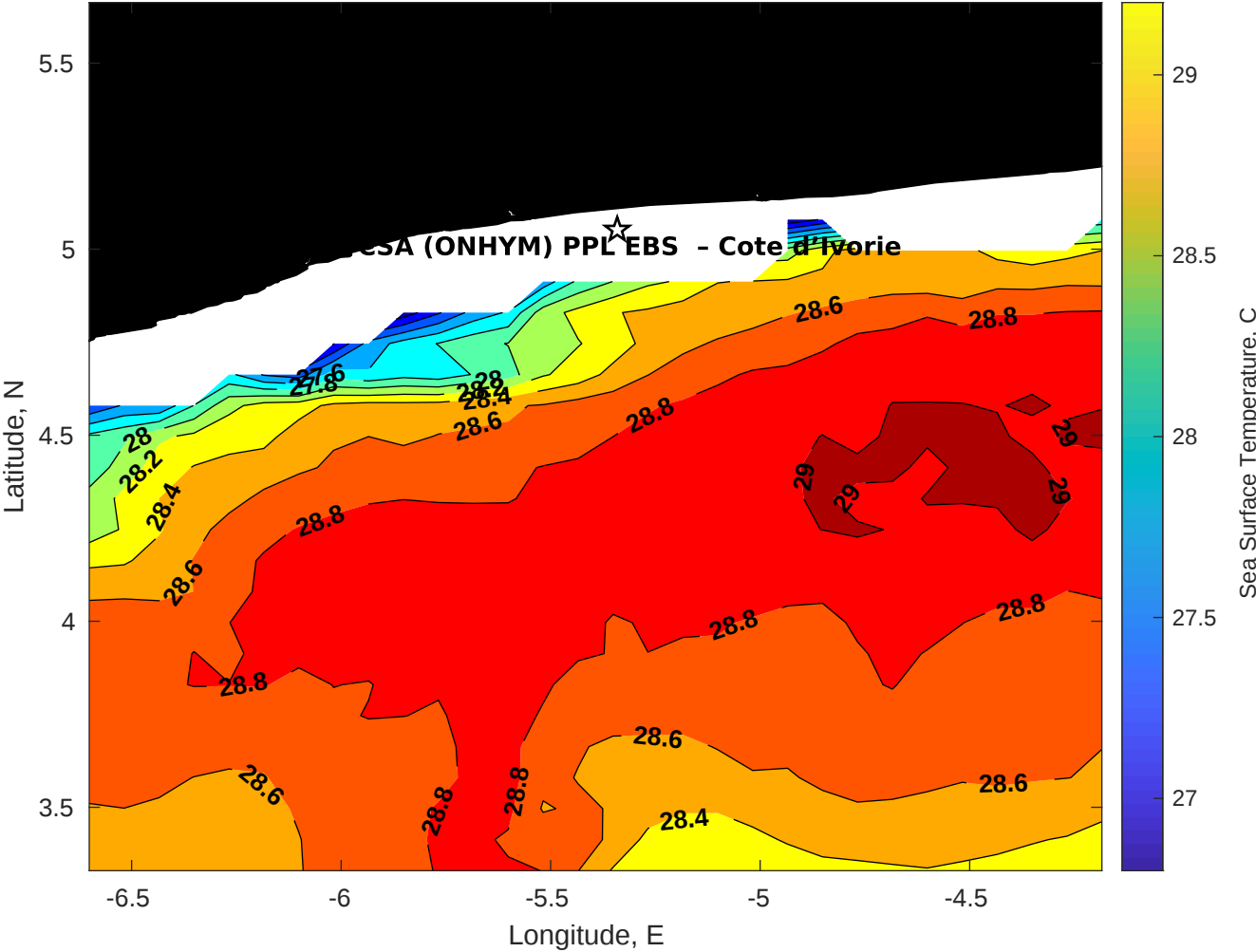
SST for CSA (ONHYM) PPL EBS - Cote d'Ivoire at 05-Dec-2025 00:00:00
