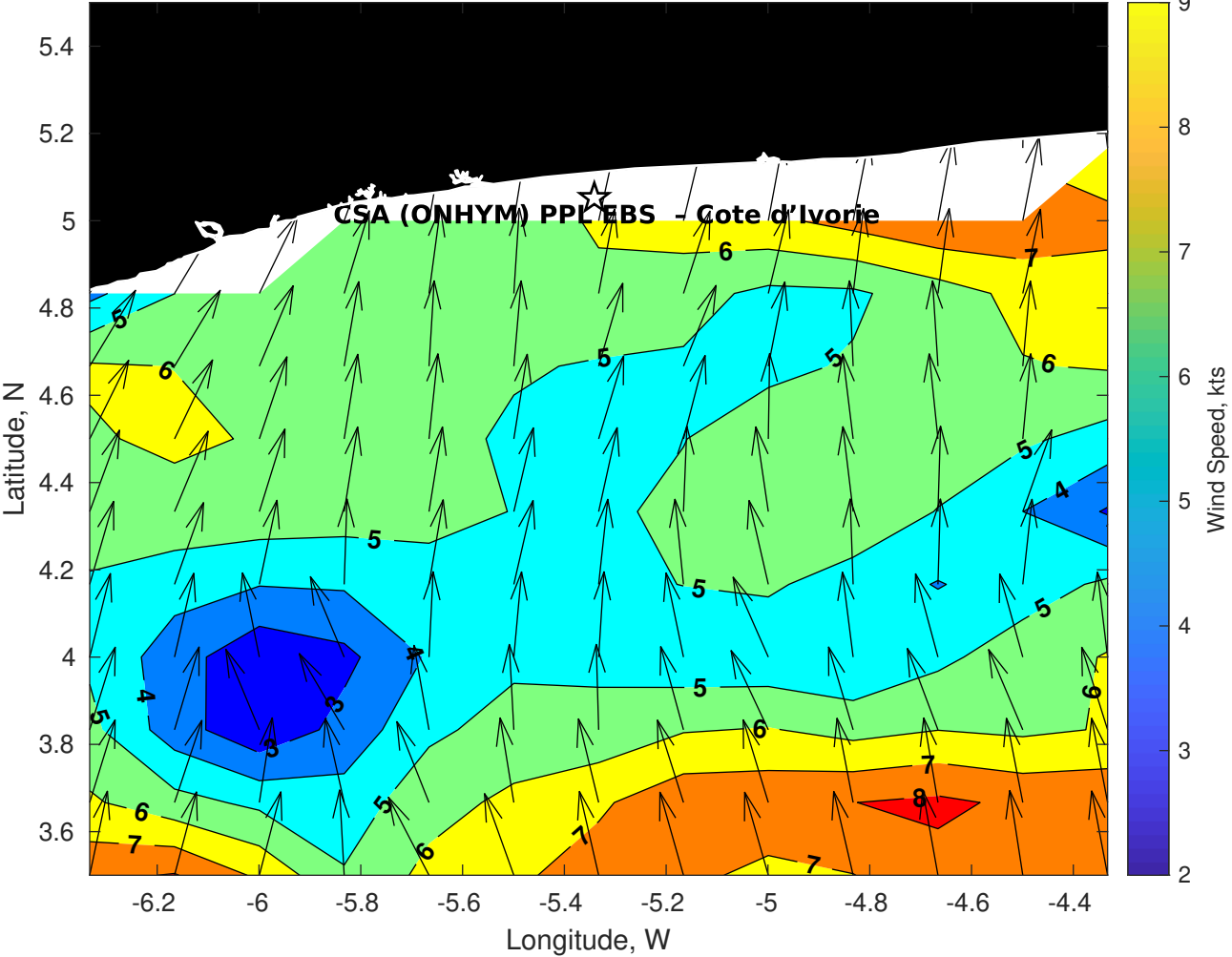
GFS Winds (kts) for CSA (ONHYM) PPL EBS - Cote d'Ivoire at 06-Dec-2025 09:00:00
