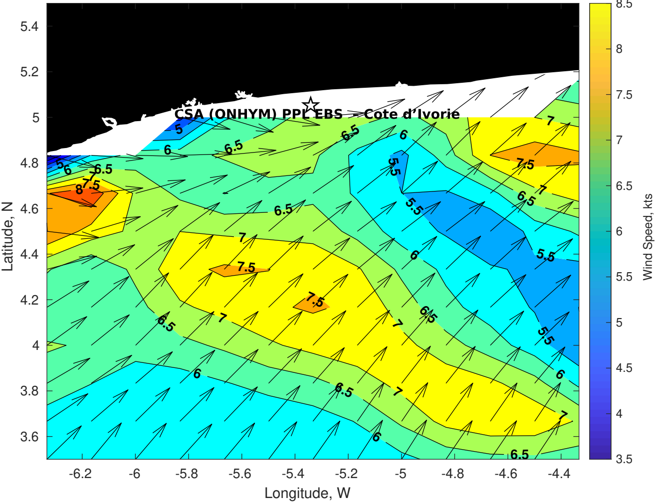
GFS Winds (kts) for CSA (ONHYM) PPL EBS - Cote d'Ivoire at 07-Dec-2025 09:00:00
