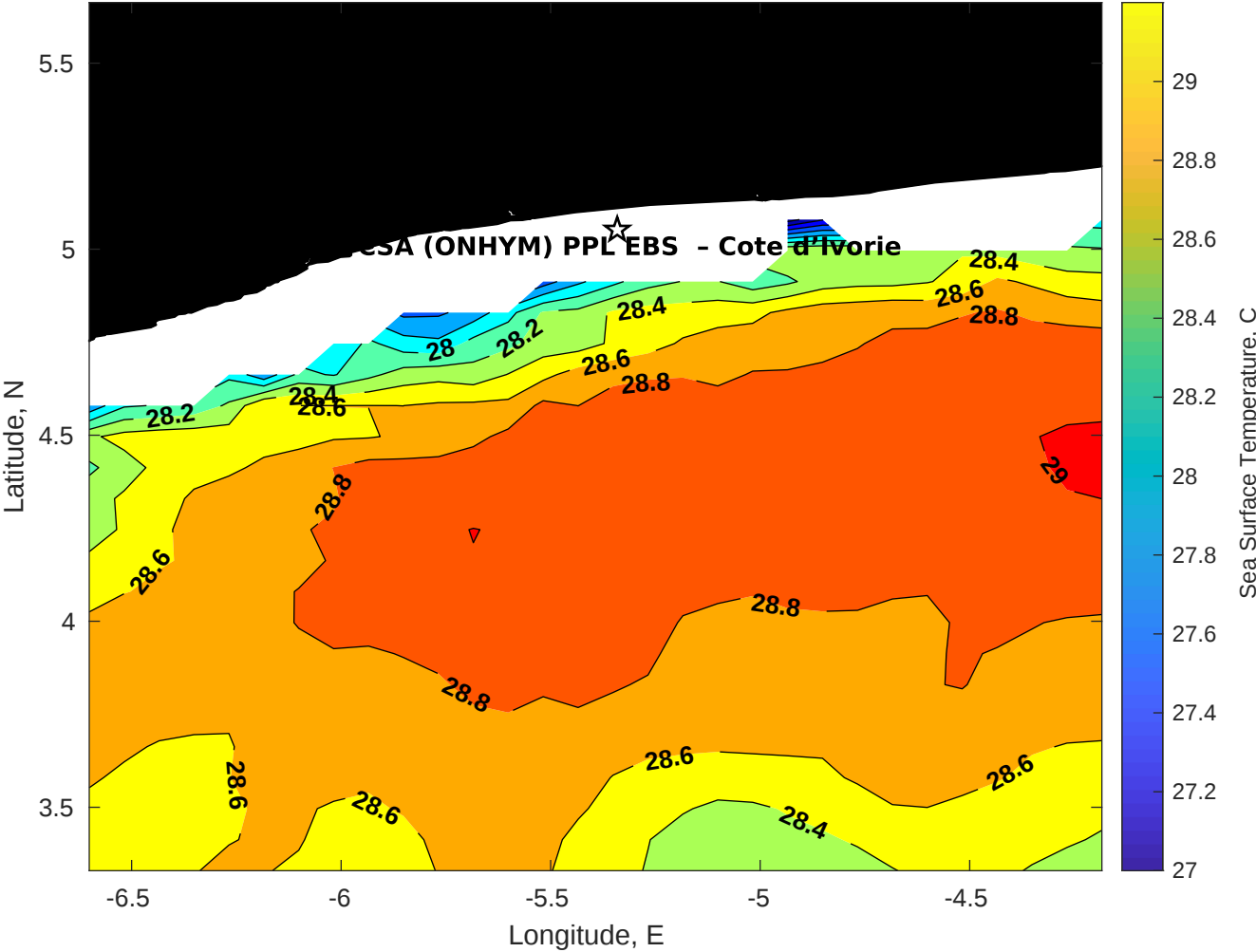
SST for CSA (ONHYM) PPL EBS - Cote d'Ivoire at 07-Dec-2025 00:00:00
