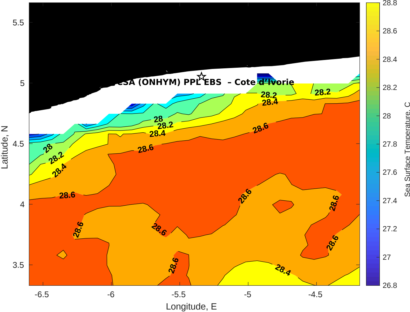
SST for CSA (ONHYM) PPL EBS - Cote d'Ivoire at 08-Dec-2025 00:00:00
