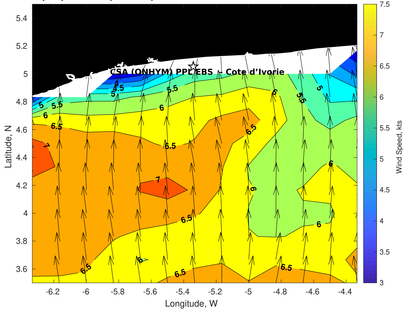
GFS Winds (kts) for CSA (ONHYM) PPL EBS - Cote d'Ivoire at 10-Dec-2025 09:00:00
