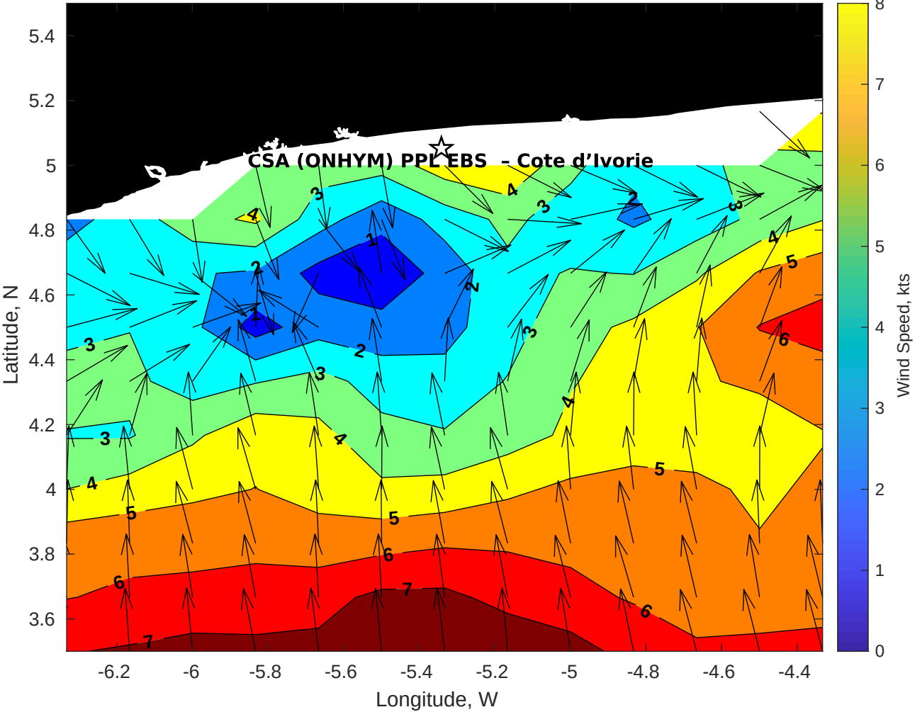
GFS Winds (kts) for CSA (ONHYM) PPL EBS - Cote d'Ivoire at 16-Dec-2025 09:00:00
