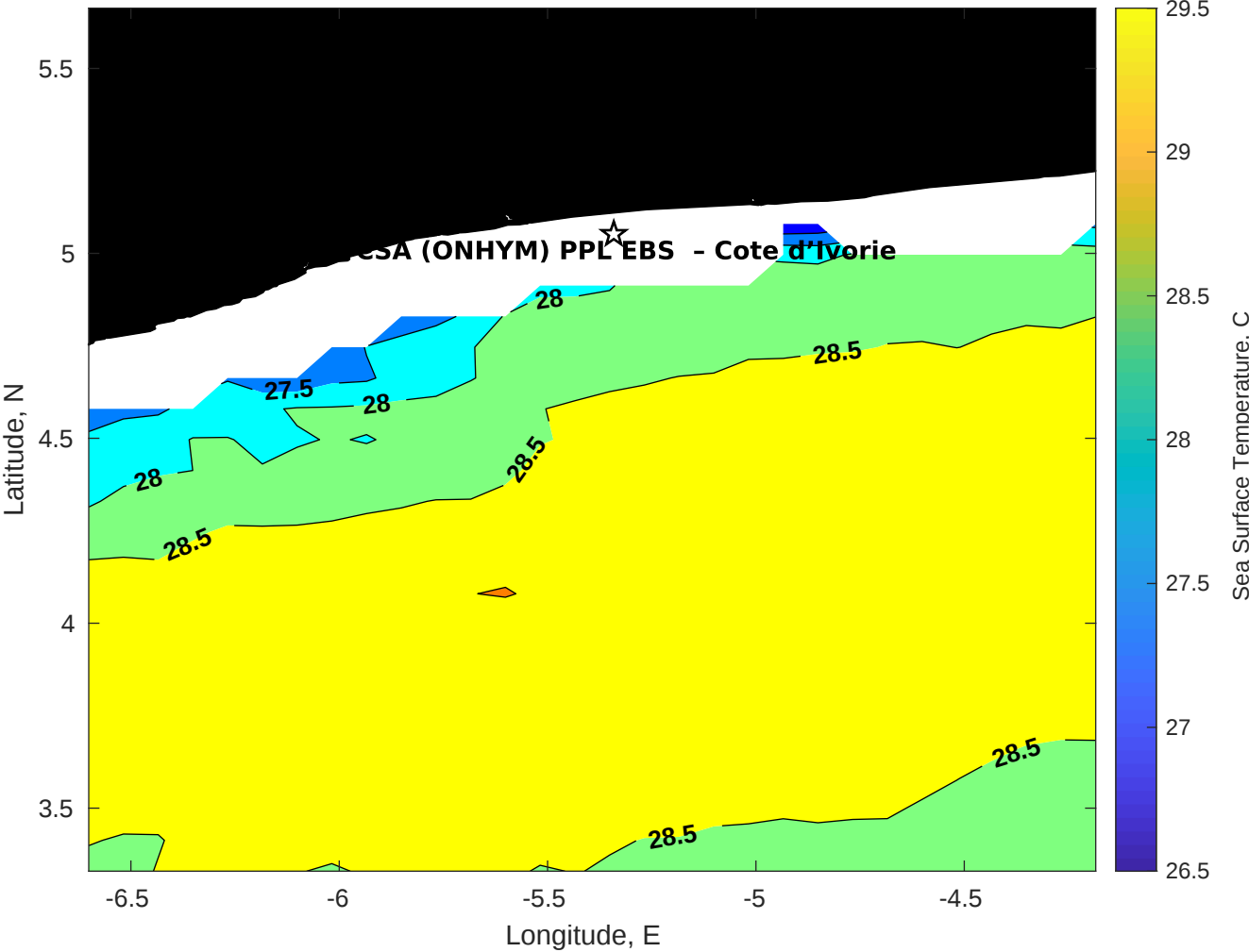
SST for CSA (ONHYM) PPL EBS - Cote d'Ivoire at 16-Dec-2025 00:00:00
