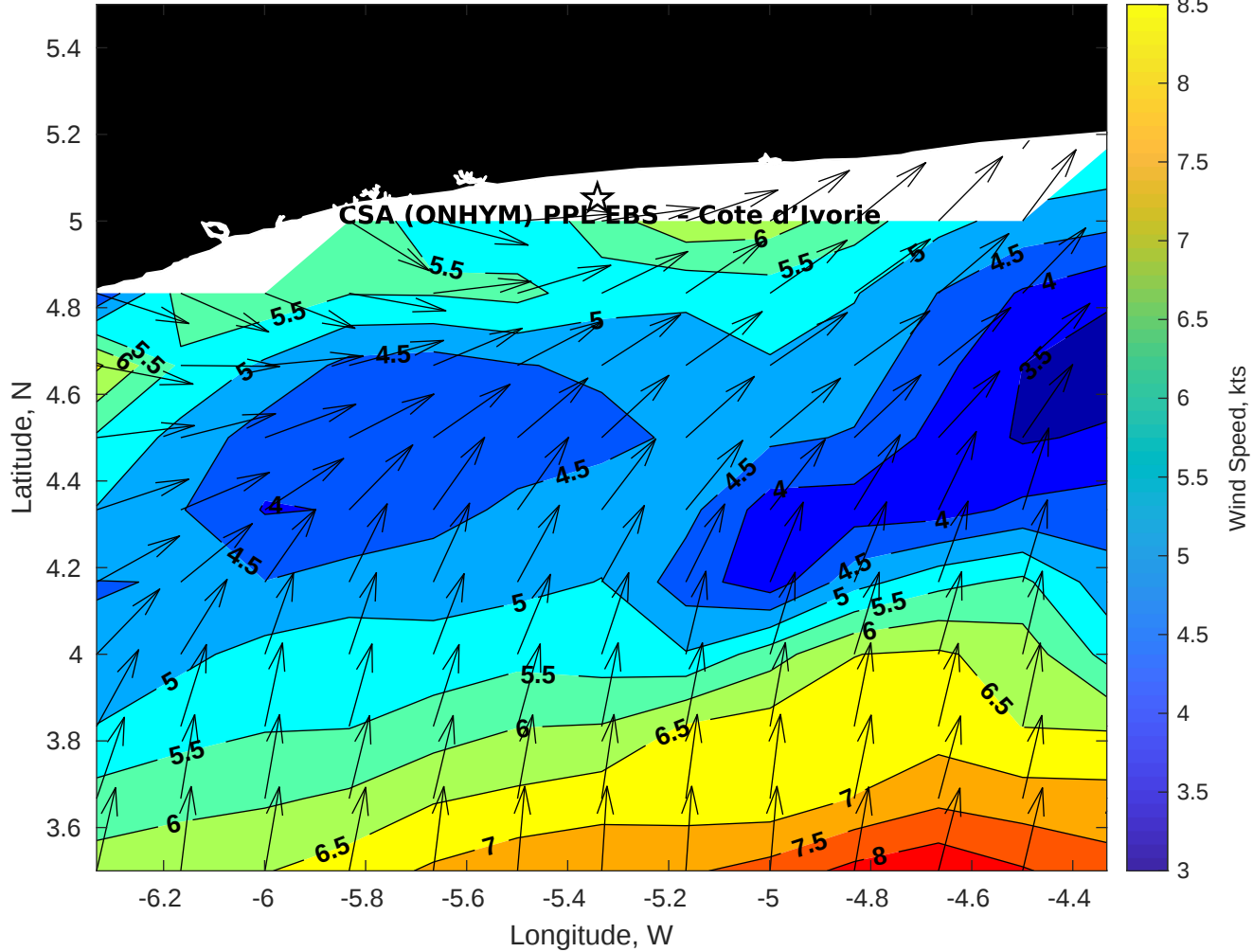
GFS Winds (kts) for CSA (ONHYM) PPL EBS - Cote d'Ivoire at 17-Dec-2025 09:00:00
