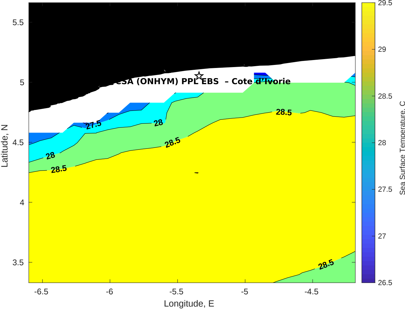
SST for CSA (ONHYM) PPL EBS - Cote d'Ivoire at 17-Dec-2025 00:00:00
