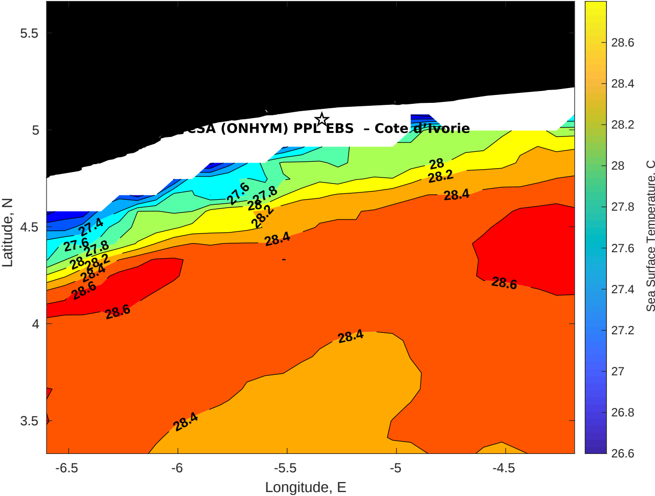
SST for CSA (ONHYM) PPL EBS - Cote d'Ivoire at 20-Dec-2025 00:00:00
