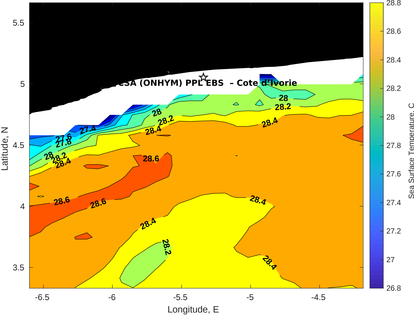
SST for CSA (ONHYM) PPL EBS - Cote d'Ivoire at 22-Dec-2025 00:00:00
