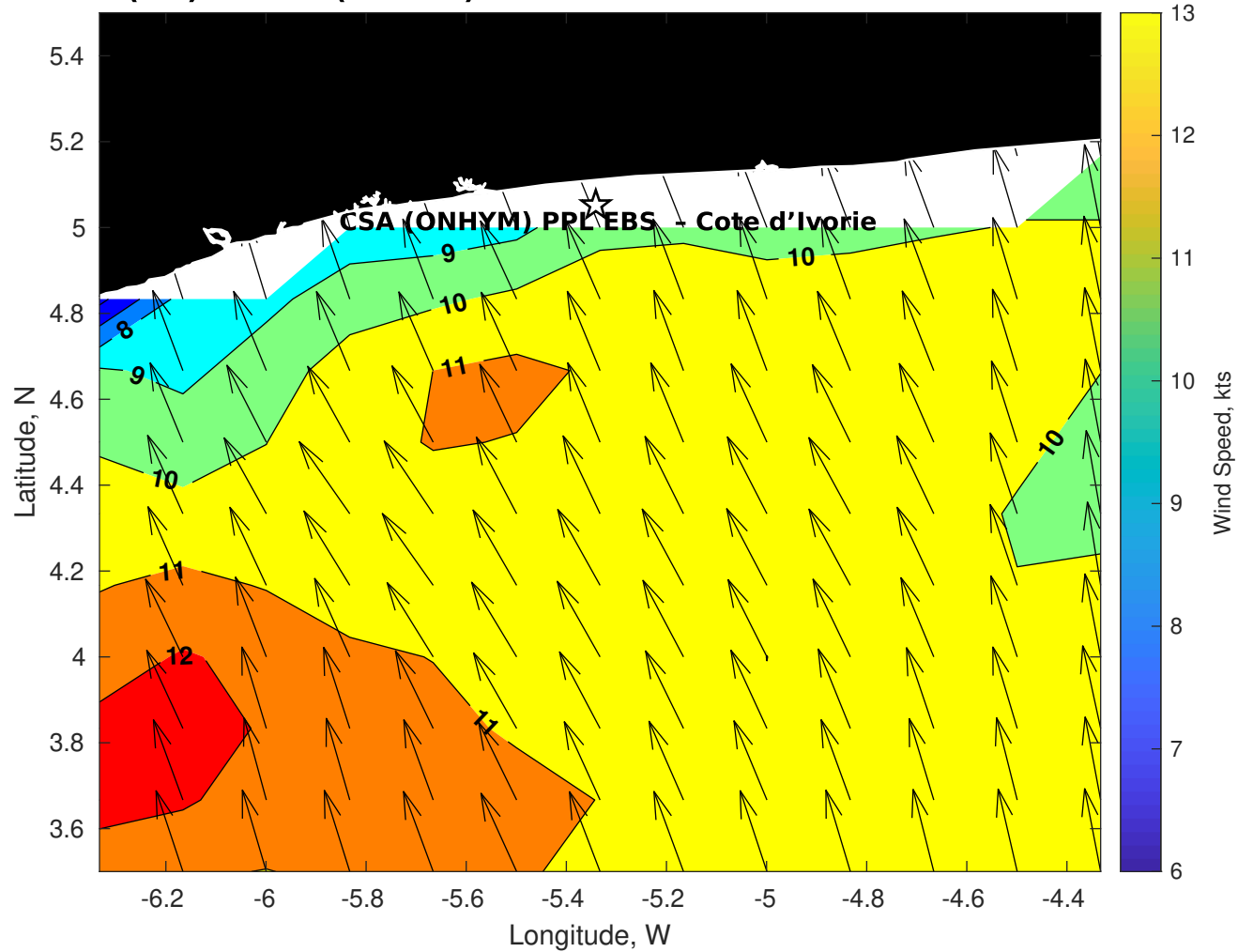
GFS Winds (kts) for CSA (ONHYM) PPL EBS - Cote d'Ivoire at 26-Dec-2025 09:00:00
