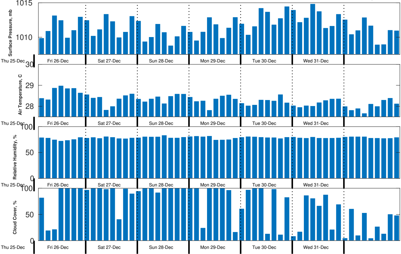
Met Forecast for CSA (ONHYM) PPL EBS - Cote d'Ivoire from 26-Dec-2025 00:00:00 to 02-Jan-2026 00:00:00
