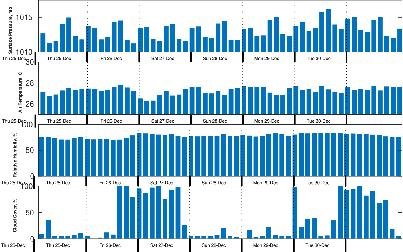
Met Forecast for Gyre from 25-Dec-2025 20:00:00 to 01-Jan-2026 20:00:00
