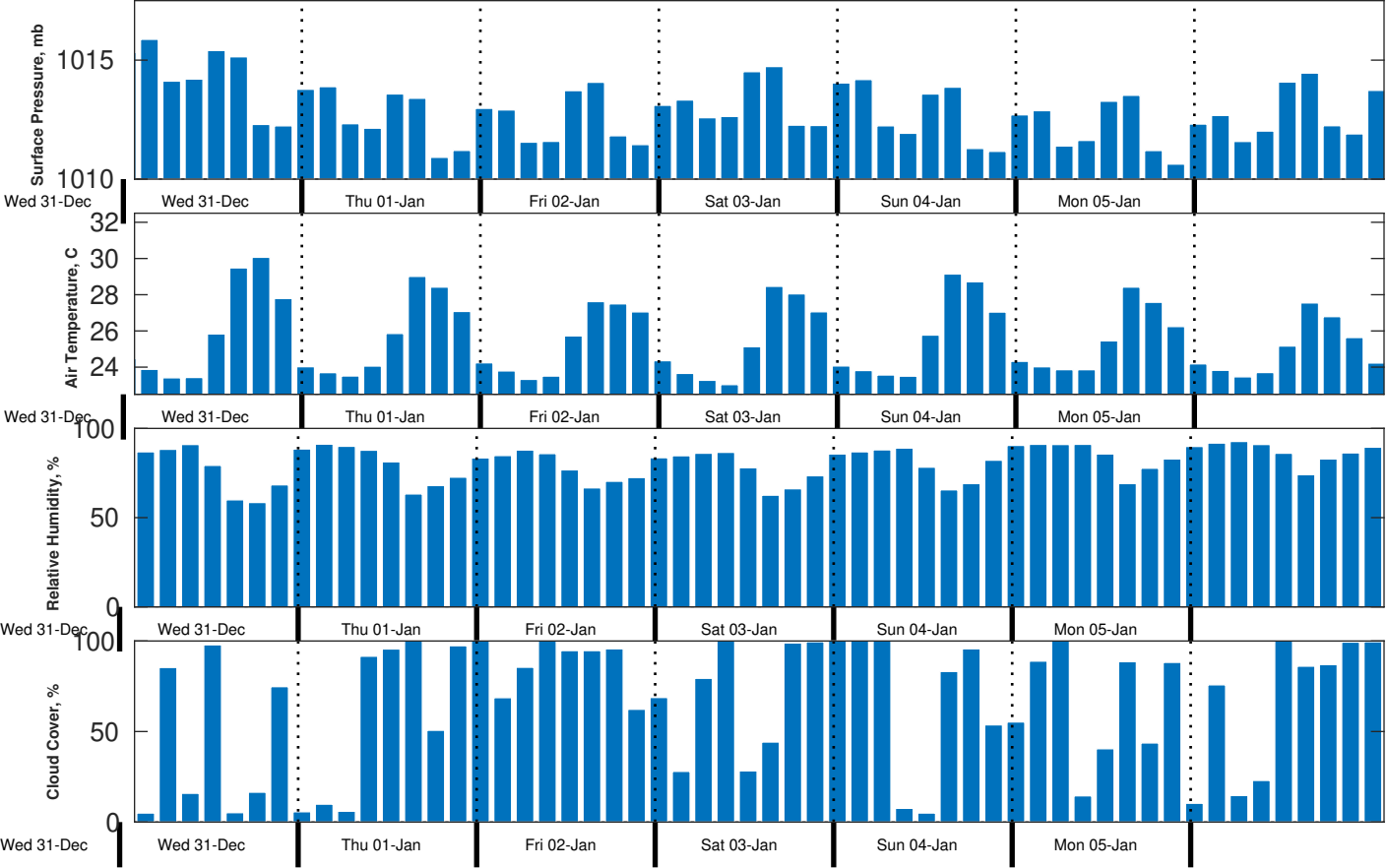
Met Forecast for Gyre from 31-Dec-2025 20:00:00 to 07-Jan-2026 20:00:00
