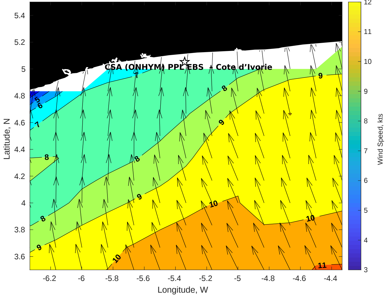
GFS Winds (kts) for CSA (ONHYM) PPL EBS - Cote d'Ivoire at 03-Jan-2026 09:00:00
