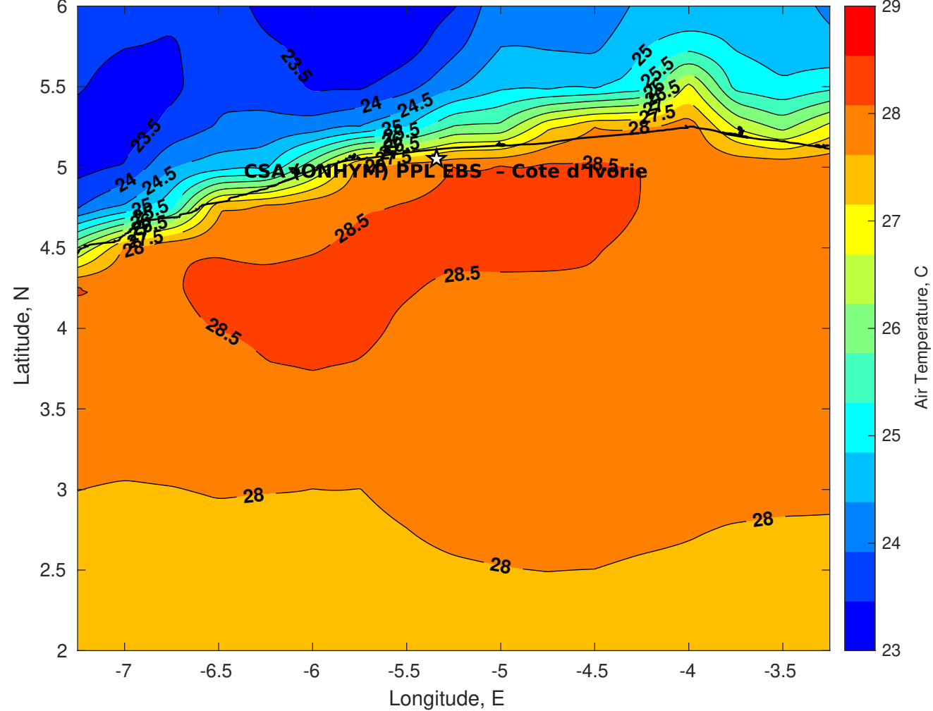
Air Temperature (C) for CSA (ONHYM) PPL EBS - Cote d'Ivoire at 03-Jan-2026
