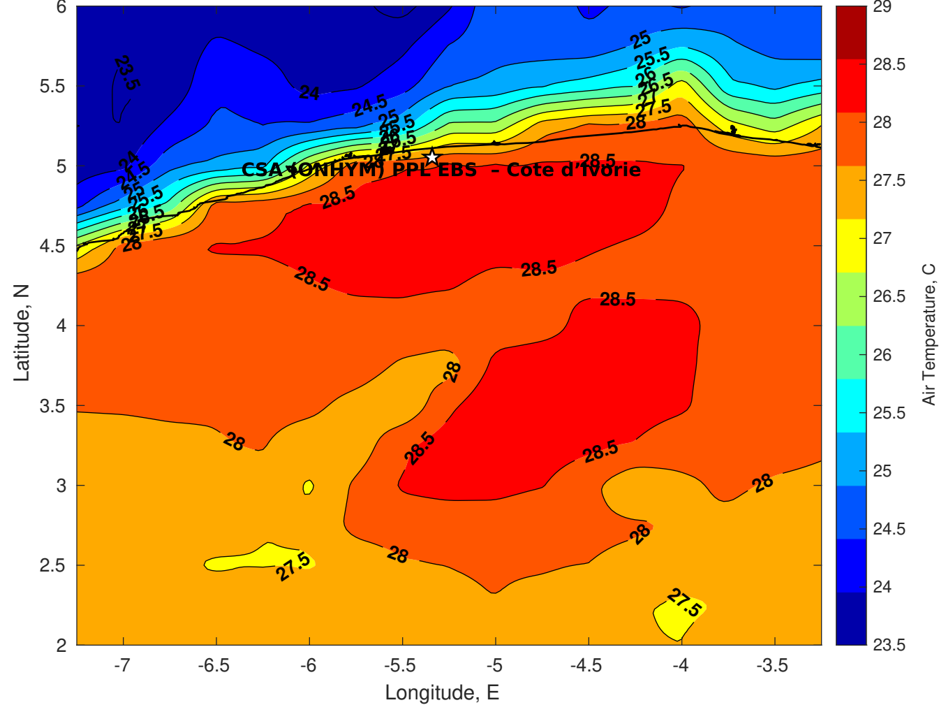
Air Temperature (C) for CSA (ONHYM) PPL EBS - Cote d'Ivoire at 03-Jan-2026
