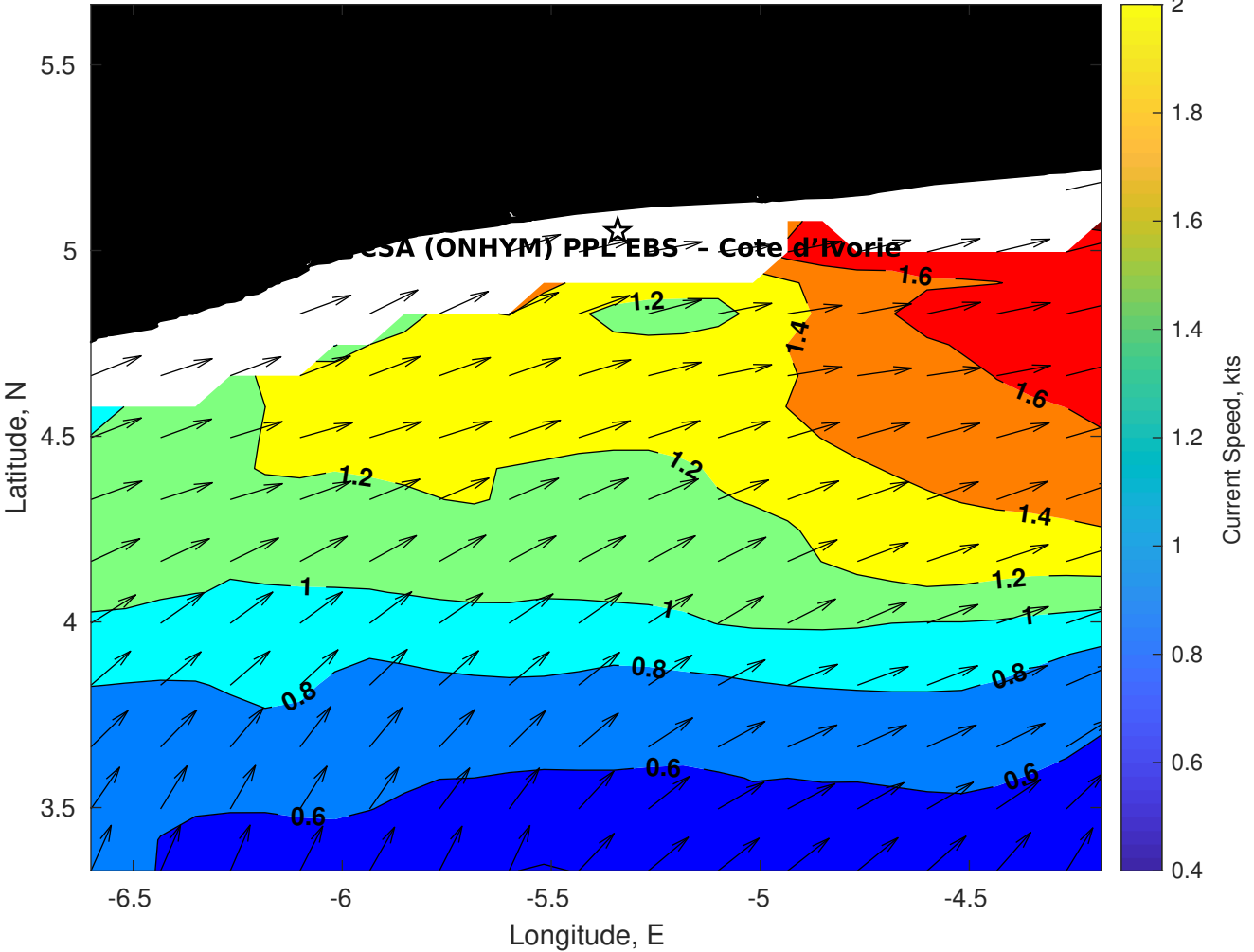
Surface Currents for CSA (ONHYM) PPL EBS - Cote d'Ivoire at 02-Jan-2026 00:00:00
