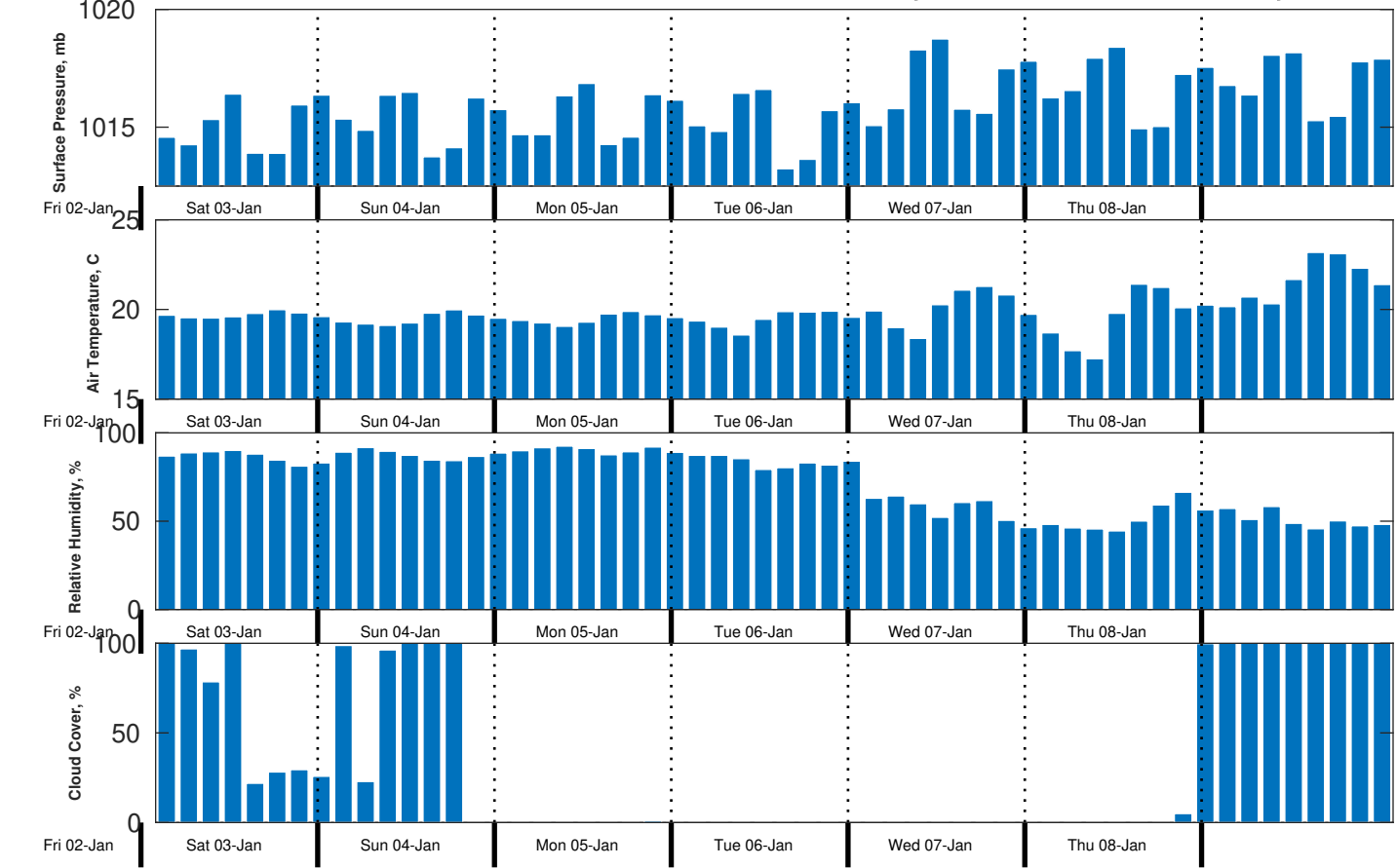
Met Forecast for CSA (ONHYM) PPL EBS - Mauritania from 03-Jan-2026 00:00:00 to 10-Jan-2026 00:00:00
