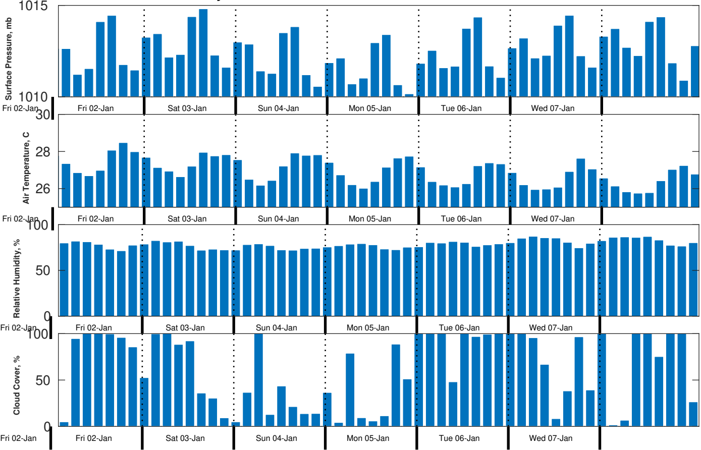
Met Forecast for Gyre from 02-Jan-2026 20:00:00 to 09-Jan-2026 20:00:00
