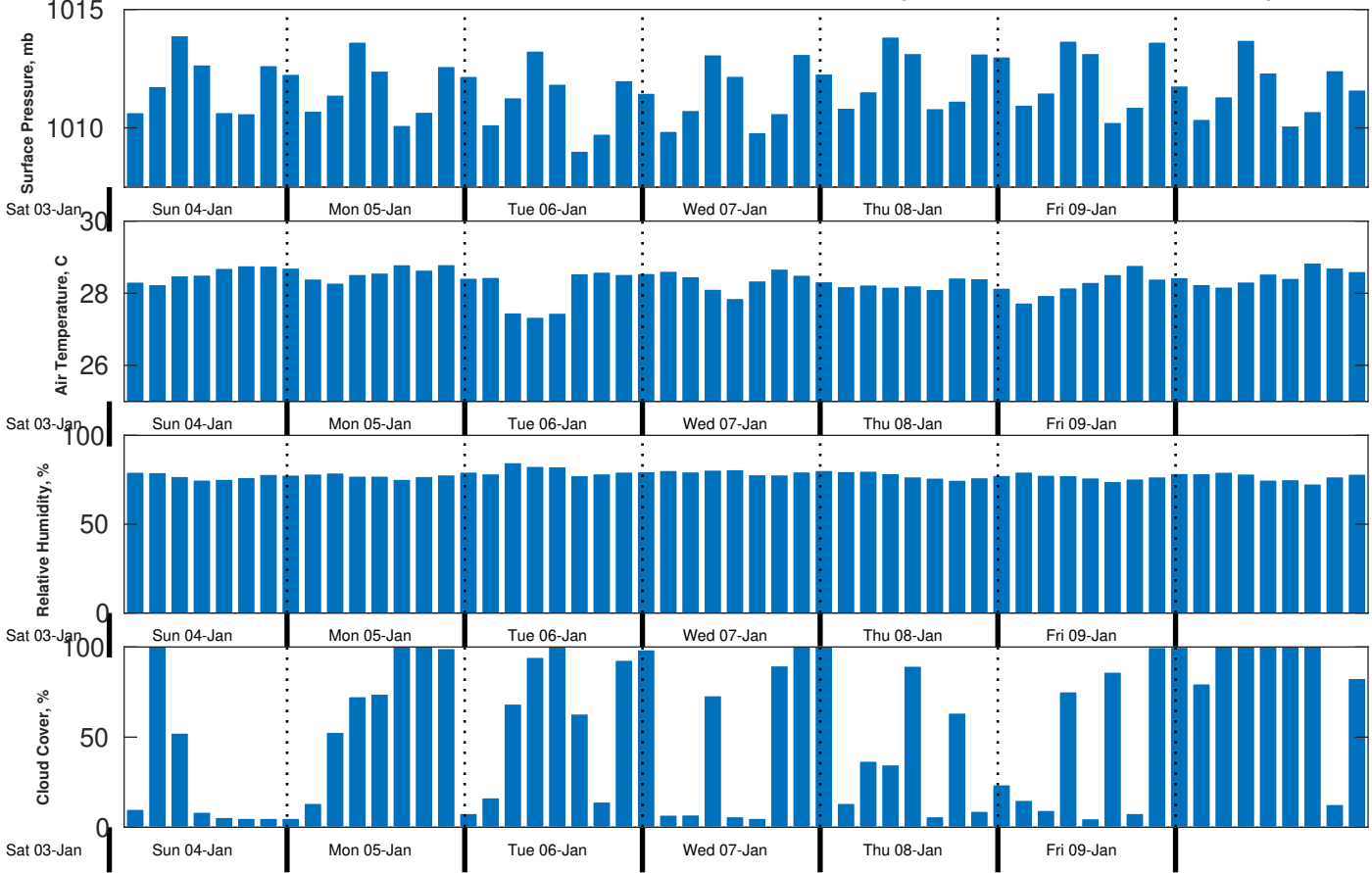
Met Forecast for CSA (ONHYM) PPL EBS - Cote d'Ivoire from 04-Jan-2026 00:00:00 to 11-Jan-2026 00:00:00
