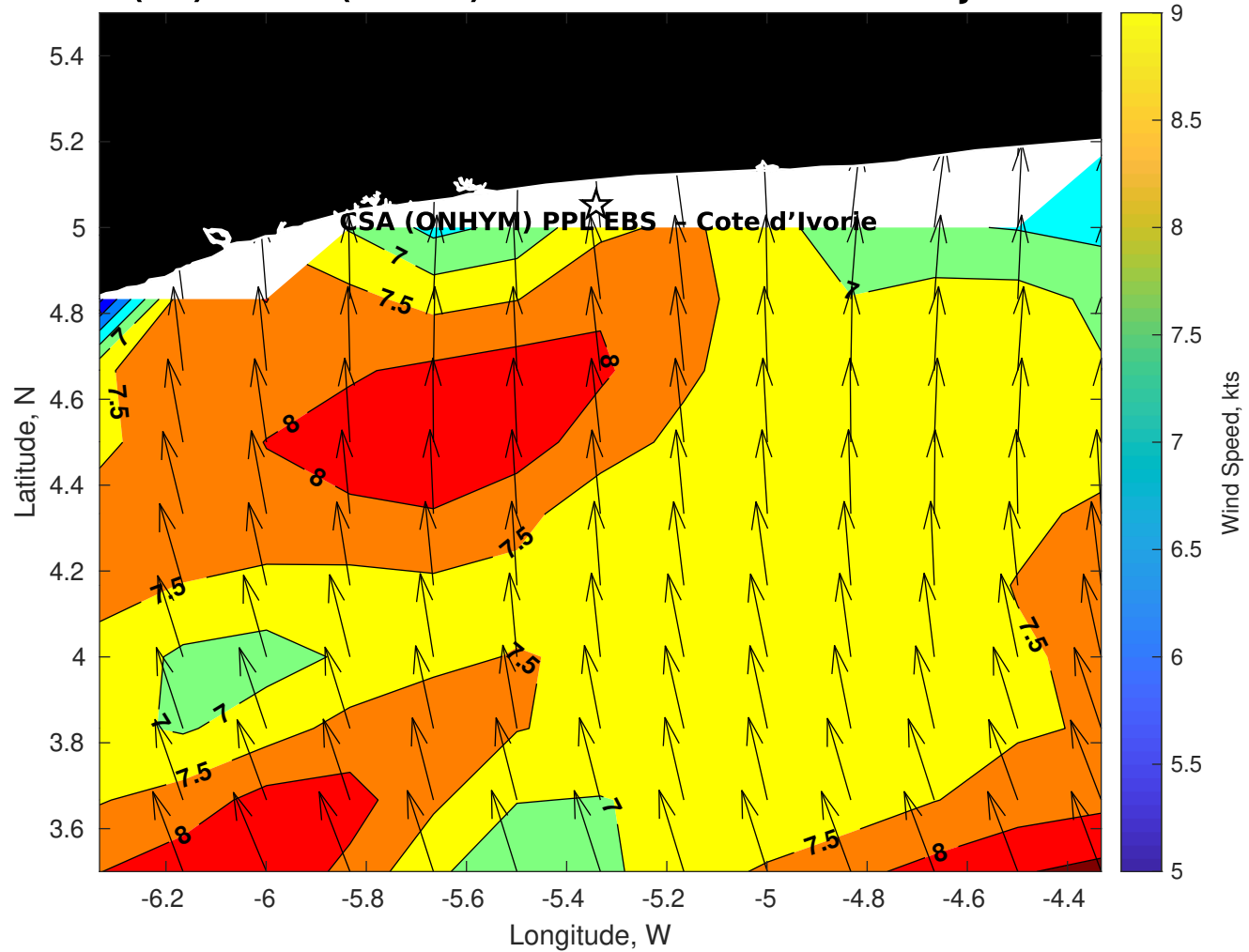
GFS Winds (kts) for CSA (ONHYM) PPL EBS - Cote d'Ivoire at 04-Jan-2026 09:00:00
