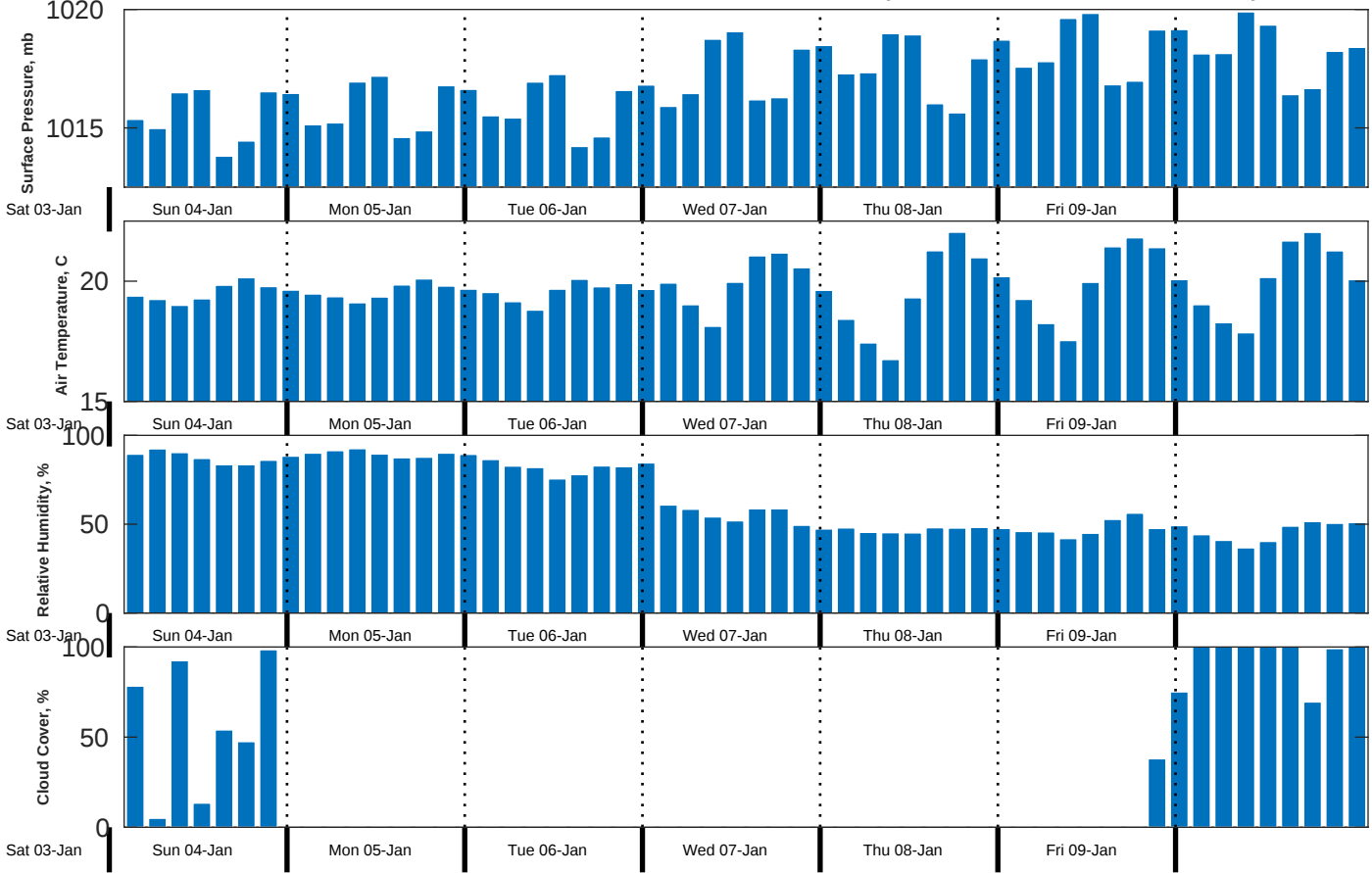
Met Forecast for CSA (ONHYM) PPL EBS - Mauritania from 04-Jan-2026 00:00:00 to 11-Jan-2026 00:00:00
