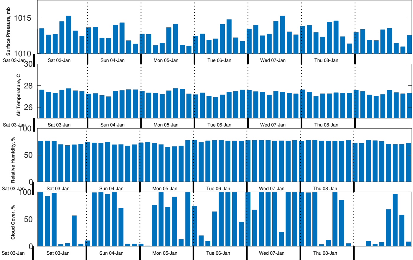
Met Forecast for Gyre from 03-Jan-2026 20:00:00 to 10-Jan-2026 20:00:00
